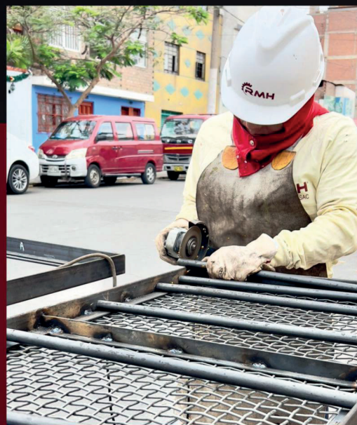
Fabricación integral de rejillas metálicas
